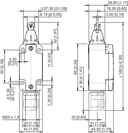
Rollenstößel 8070/2--R-U60
