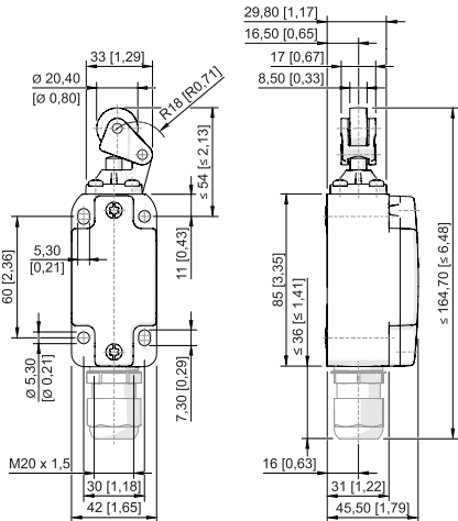
Rollenhebel 8070/2-.-WH-U60
