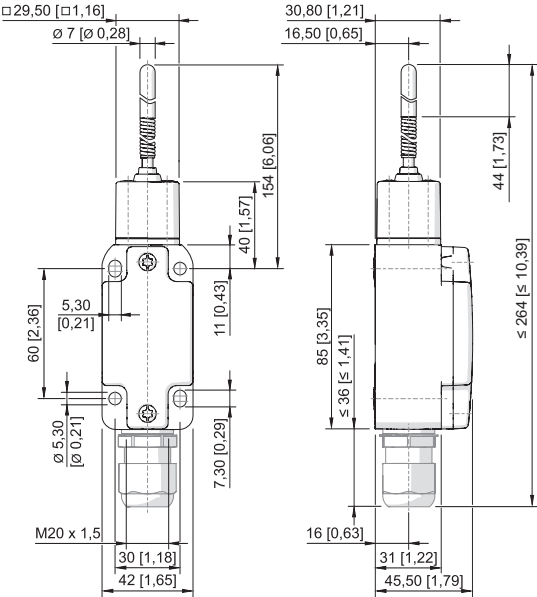
Federstab 8070/2-.-TK-U60
