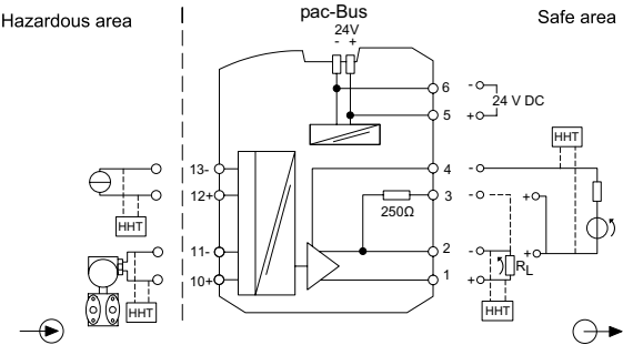
Anschlussbild 9260/13-11-10
