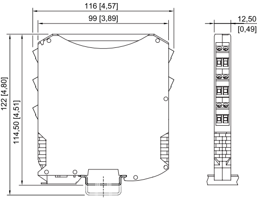
ISpac Reihen 9260, 9270, 9275, 9276, 9282 mit Federzugklemme
