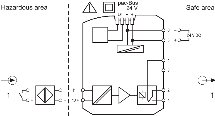
Anschlussbild 9270/11-16-14
