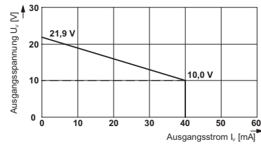
Ausgangskennlinie 9276/10-21-40
