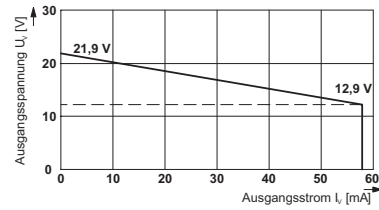
Ausgangskennlinie 9276/10-21-60-00
