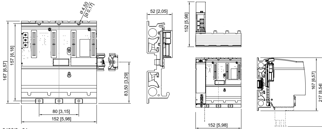
CPU Module 9442/35 + Sockel 9496/35-04-00
