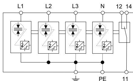
Typ 8530/1-SPD-STD1-2-TNS-ACI-3LN2
