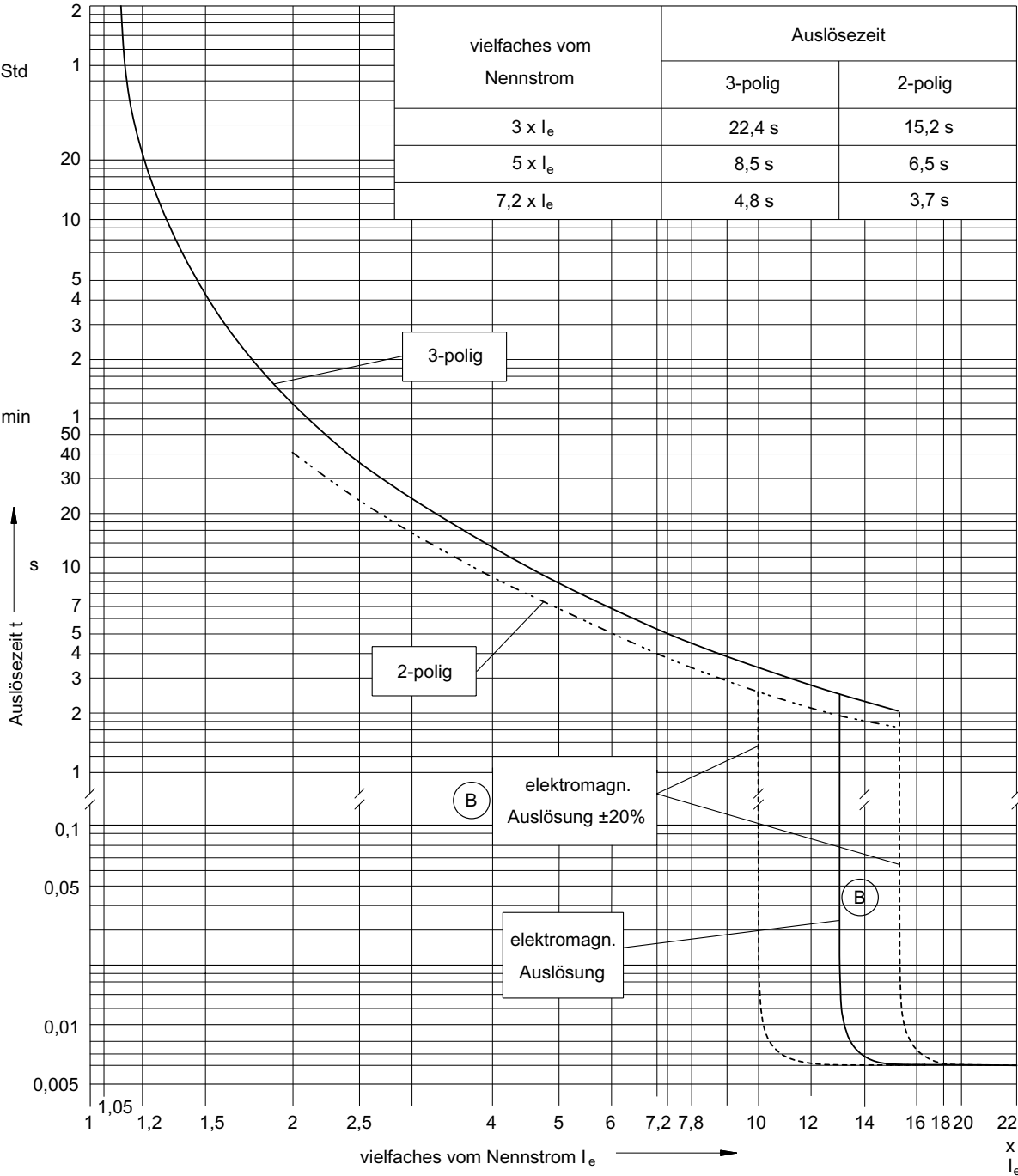
Auslösekennlinie 4 ... 6,3 A
