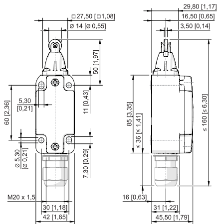
Rollenstößel 8070/2--R-U60
