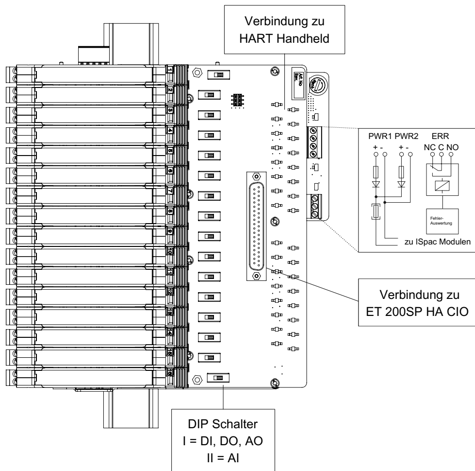
Anschlussbild 9295/21AH-SI3-01A5
