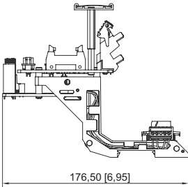
Maßzeichnung (alle Maße in mm [Zoll]) – Änderungen vorbehalten
