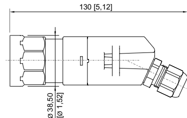
8003/...-010, 8003/...-012 Pilzsperrtaster Ø 38 mm
