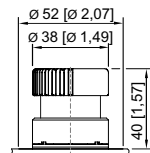
8003/...-010, 8003/...-012 Pilzsperrtaster Ø 38 mm
