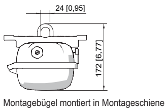
Montageschiene
