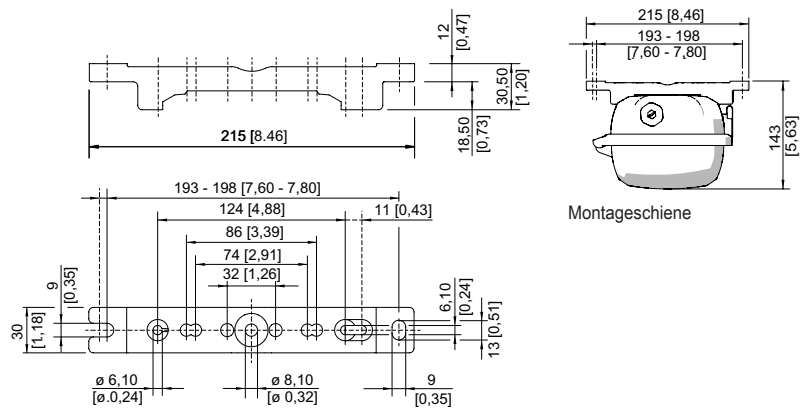
Montageschiene
