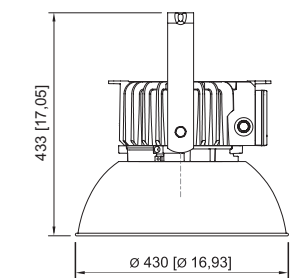
Mit Montagebügel
