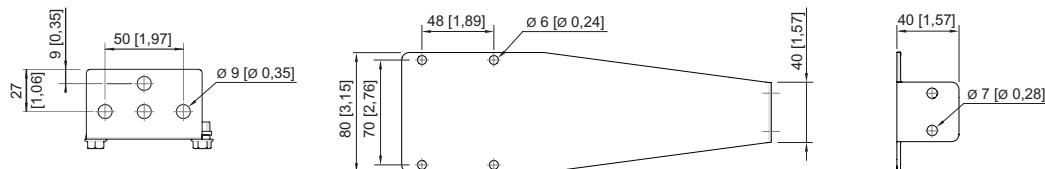
Montageklammer Gewinde
