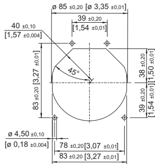
Flanschsteckdose 4-/5-polig Öffnungsbild
