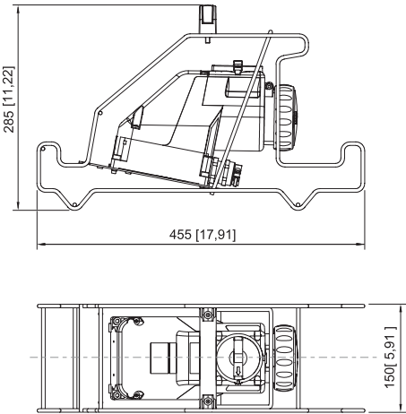
Kupplungsdose
