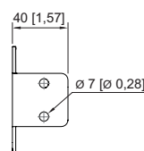
Montageklammer Gewinde
