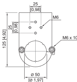
Montageklammer Fläche
