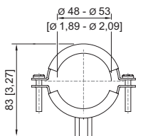
Montageklammer Gewinde
