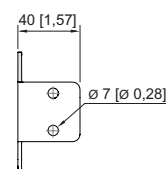
Montageklammer Gewinde
