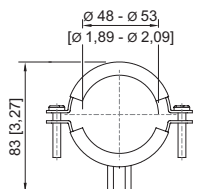
Montageklammer Gewinde
