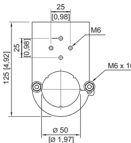
Montageklammer Fläche
