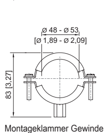
Montageklammer Gewinde
