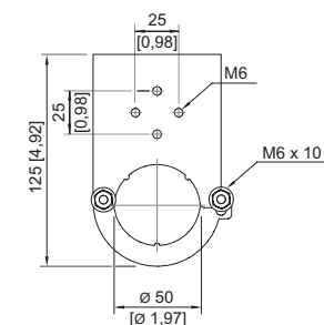
Montageklammer Fläche
