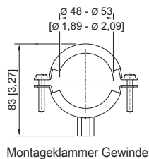
Montageklammer Gewinde
