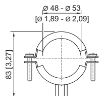
Montageklammer Gewinde
