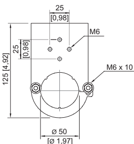
Montageklammer Fläche
