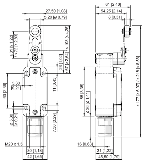
Schwenkhebel 8070/2-5-DS-U60
