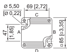
8118/.1. Enclosure SZ 1
