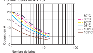
Intensité du courant des câbles 1,5 mm 2 dans M24 x 1,5
