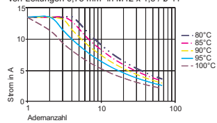
Strombelastbarkeit von Leitungen 0,75 mm 2 in M42 x 1,5 / ø 41
