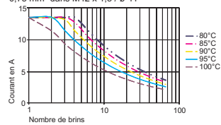
Intensité du courant des câbles 0,75 mm 2 dans M42 x 1,5 / ø 41
