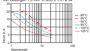
Strombelastbarkeit von Leitungen 1,5 mm 2 in M33 x 1,5 / ø 34
