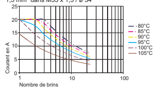
Intensité du courant des câbles 1,5 mm 2 dans M33 x 1,5 / ø 34
