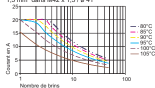
Intensité du courant des câbles 1,5 mm 2 dans M42 x 1,5 / ø 41
