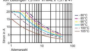
Strombelastbarkeit von Leitungen 1,5 mm 2 in M42 x 1,5 / ø 41
