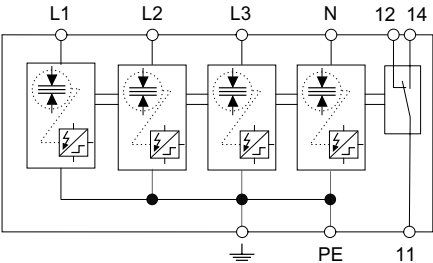
Type 8530/1-SPD-STD1-2-TNS-ACI-3LN2
