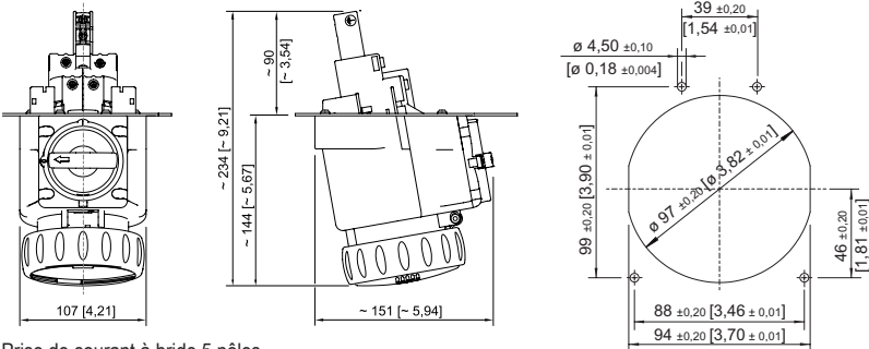
Prise de courant à bride 5 pôles Position horaire 5 h, 6 h, 7 h
