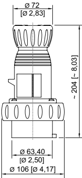
Fiche 5 pôles
