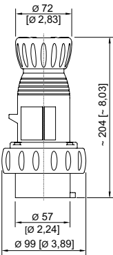
Fiche 4 pôles
