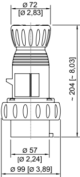
Fiche 4 pôles
