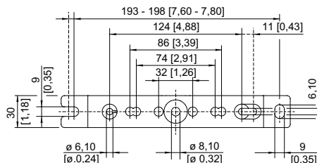
Support rail DIN
