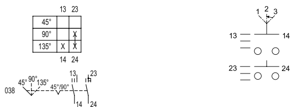
Schéma de fonctionnement 8008/-038
