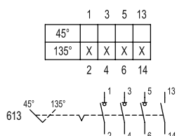
Schéma de fonctionnement 8008/-613
