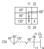
Schéma de fonctionnement 8008/-034
