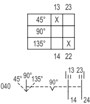
Schéma de fonctionnement 8008/2-040 Schéma de fonctionnement 8008/4-10-40
