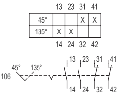
Schéma de fonctionnement 8008/2-106 Schéma de fonctionnement 8008/4-11-06
