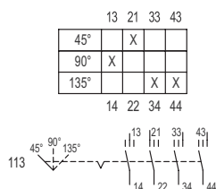
Schéma de fonctionnement 8008/-113
