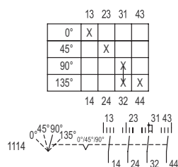
Schéma de fonctionnement 8008/-1114
